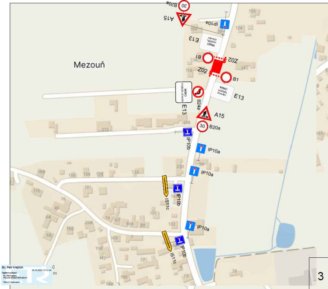
SCHEMATICKÝ PLÁNEK DO - CELKOVÁ SITUACE Uzavírka silnice III/10126 Mezouň - Nučice (Krahulov)
